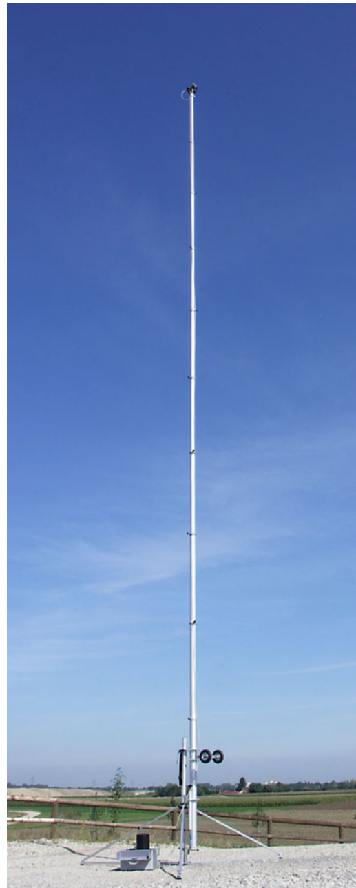
Pneumatischer Mast mit Stativstand (baugleich mit PT 75H / PT 90H / PT 105H)
