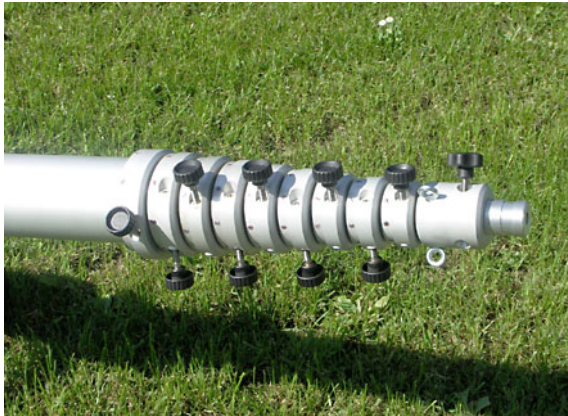
PT 75H - Stativkopf mit Feststellschrauben
